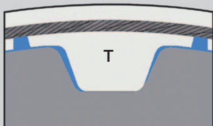
„SE“-Lücke, Reduzierte Lückenform Reduced Backlash „SE“ Tooth Gap
